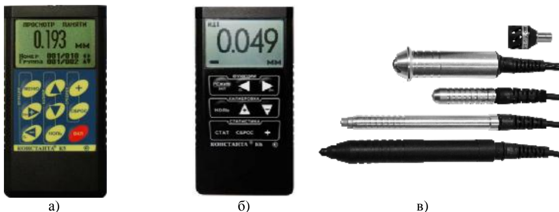
Рисунок 1 – Внешний вид а) прибор «Константа К5», б) прибор «Константа К6», в) преобразователи
